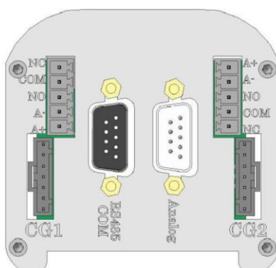
IGM402 I/O Interface
